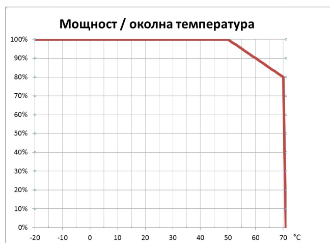
фиг. 1. Зависимост на максималната мощност от околната температура
