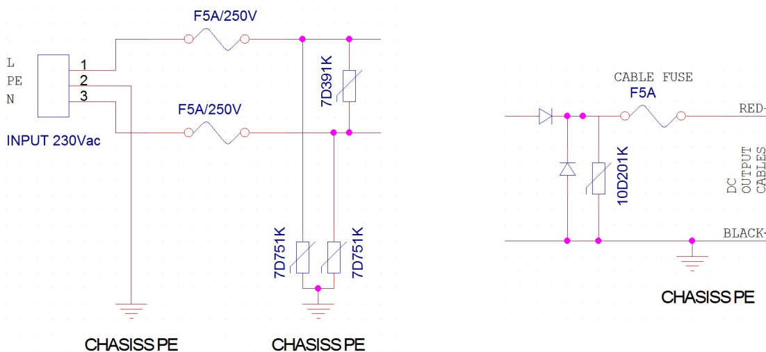
фиг. 2. Входни и изходни защитни вериги
