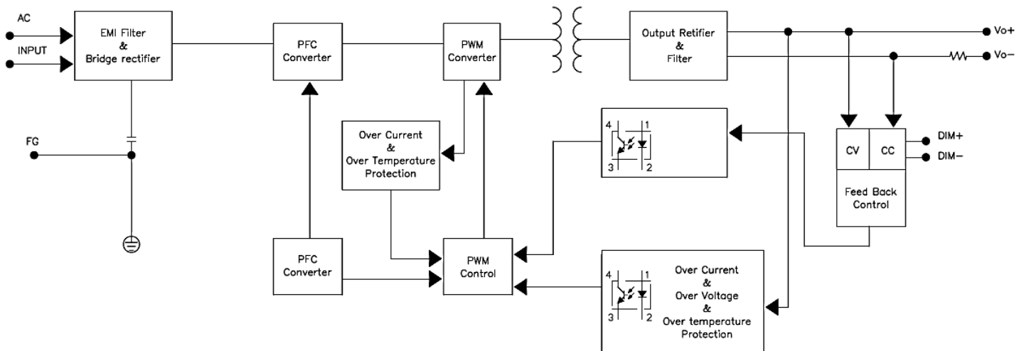
LNE-□V185WD□□
